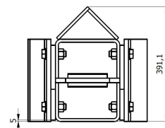
B-B ( 1:8 )
